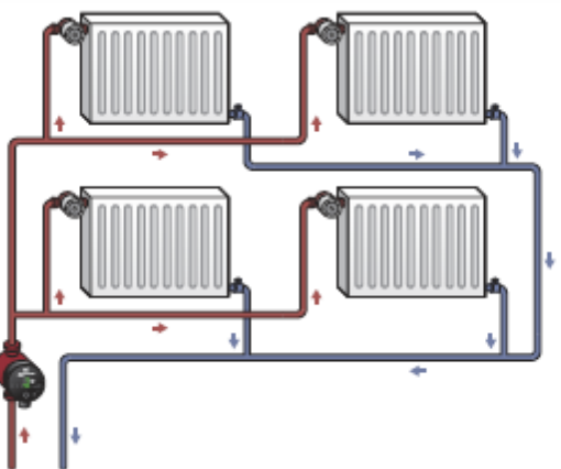
Ryc. 4 Instalacja grzewcza dwururowa
