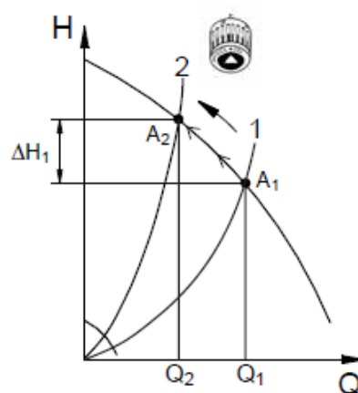
Ryc. 8 Pompa nieregulowana
