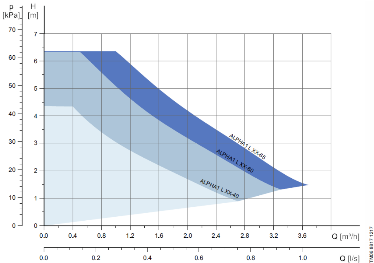
Ryc. 2 Charakterystyki (pola pracy)
