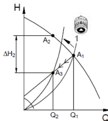
Ryc. 9 Pompa działająca w trybie proporcjonalnej regulacji ciśnienia
